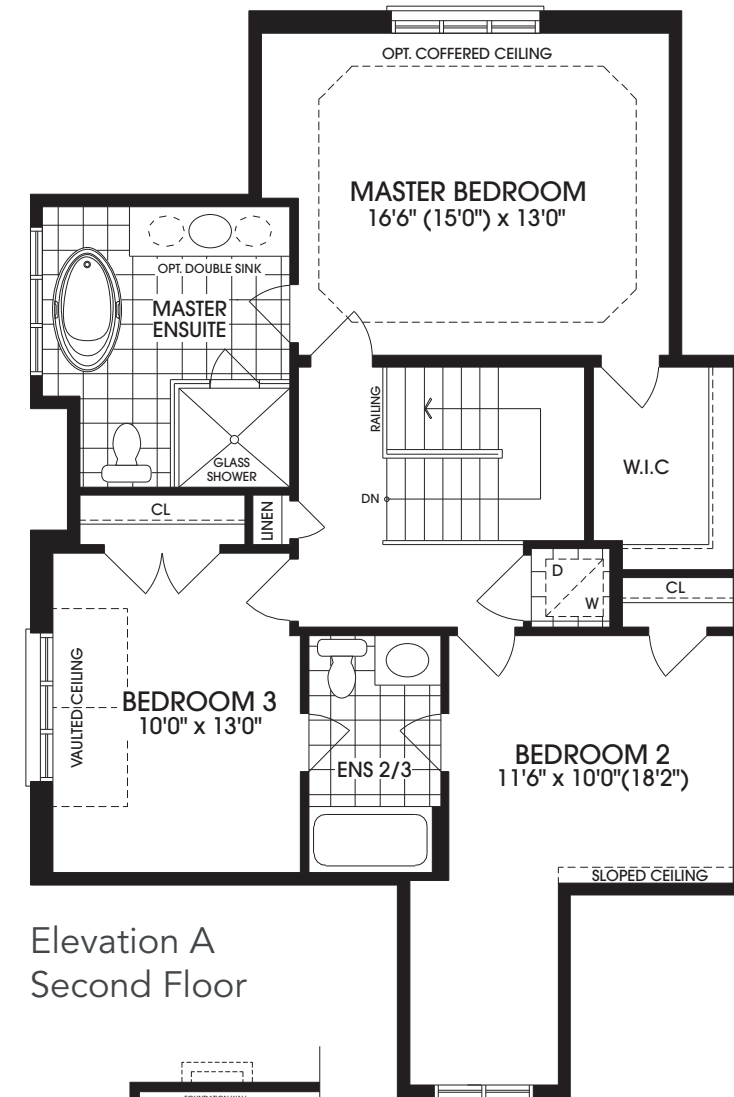
Elevation A
